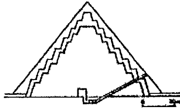
قطاع في هرم ميدوم
