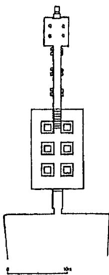
ج- تخطيط لمقبرة نبوت الثاني في أسوان.
