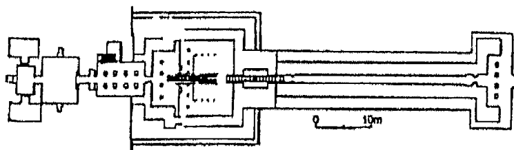
ج- تخطيط لمقبرة دواح - كا، الأول في دقاو.
