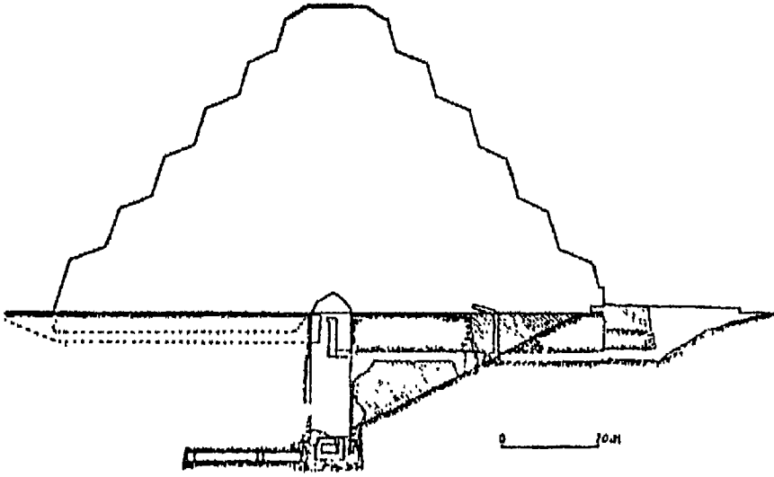
قطاع في هرم زوسر المدرج، من الشمال إلى الجنوب
